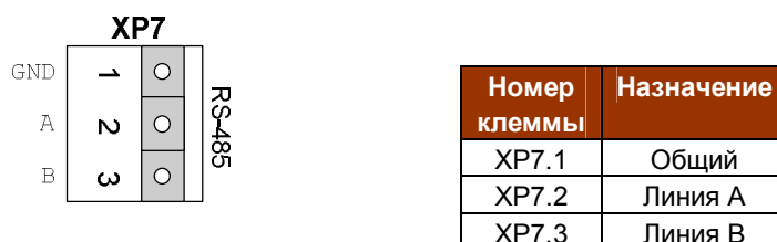
Рис. 21. Разъем XP7
