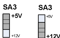
Рис. 20. Положение движкового переключателя SA3
