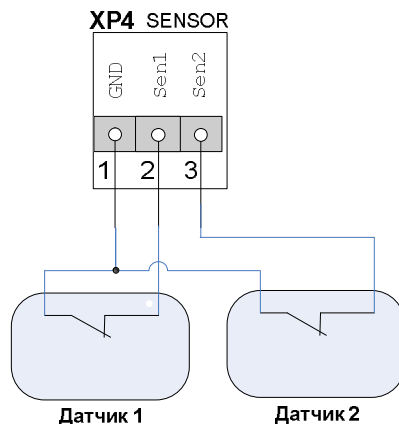
Рис. 12. Пример подключения датчиков
