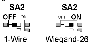
Рис. 19. Положение переключателя DIP
