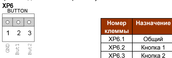
Рис. 15. Разъем XP6 (BUTTON)
