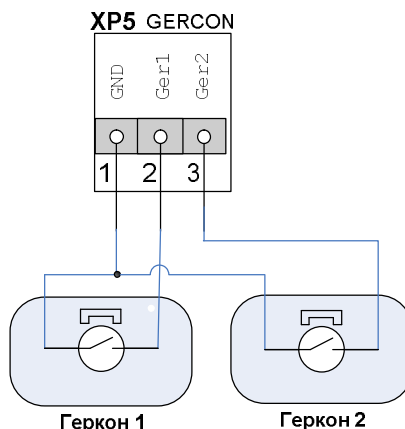
Рис. 14. Пример подключения герконов
