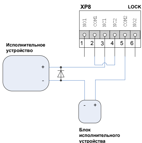
Рис. 10. Схема подключения электромагнитных замков при однодверном режиме работы контролера
