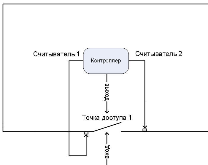
Рис. 4. Пример работы контроллера в однодверном режиме работы с функцией АВВ
