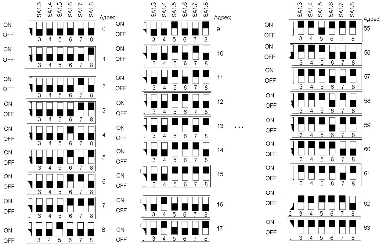
Рис. 28. Программирование сетевых адресов контроллера
