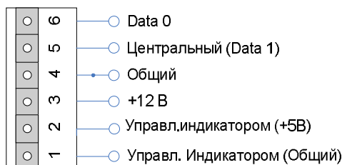
Рис. 17. Схема подключения при использовании считывателей типа «Wiegand-26»
