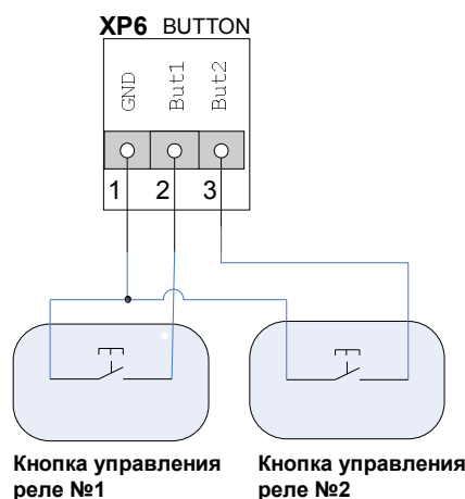
Рис. 16. Пример подключения кнопок управления реле
