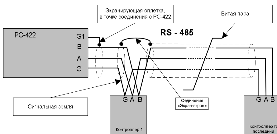
Рис. 27. Монтаж линии связи интерфейса RS-485
