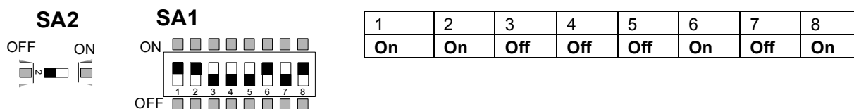
Рис. 26. Пример установки сетевого адреса «05» и скорости обмена 57600 бит/с для контроллера, не последнего в сети с однодверной конфигурацией
