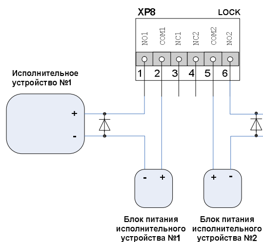
Рис. 7. Схема подключения электромеханических замков при двухдверном режиме работы контроллера
