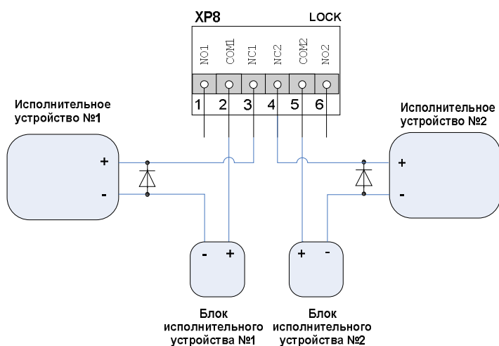
Рис. 9. Схема подключения электромагнитных замков при двухдверном режиме работы контролера
