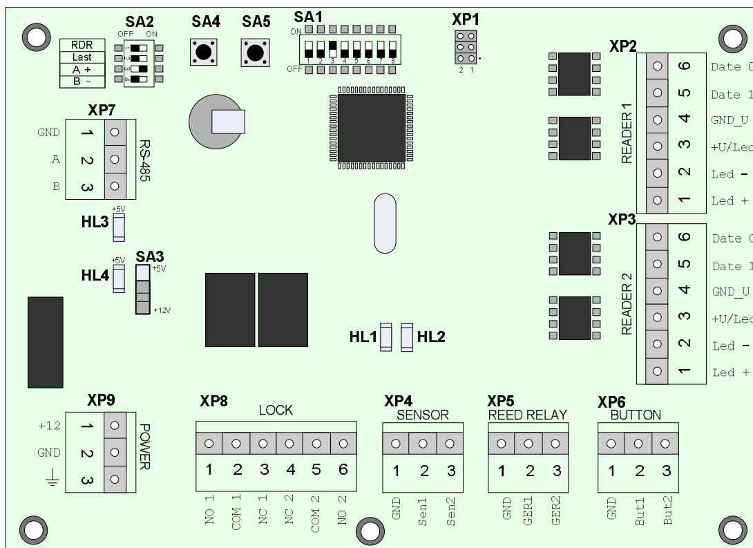
Рис. 1. Внешний вид контроллера
