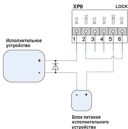
Рис. 8. Схема подключения электромеханических замков при однодверном режиме работы контроллера
